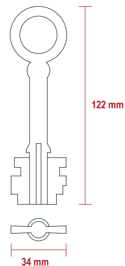
Dimensioni Chiave
