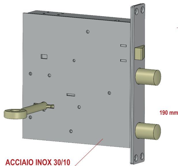
Dimensioni Serratura
